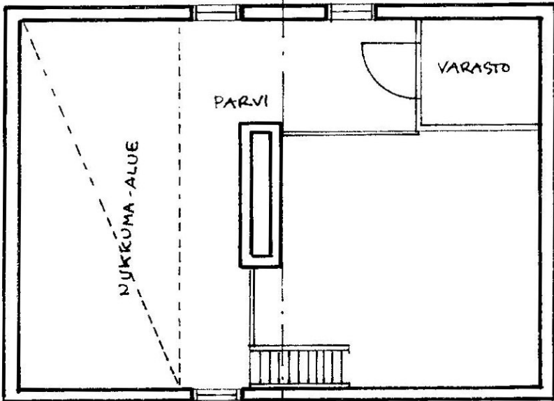
Uuden saunarakennuksen pohjapiirustus, yllä alakerta ja alla parvikerros.
